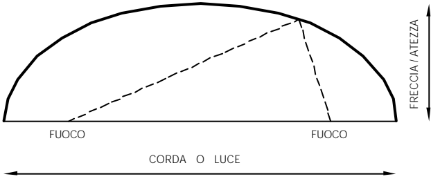
ARCO A SESTO ELLITICO
