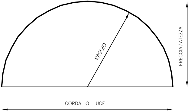
ARCO A TUTTO SESTO O A CENTRO PIENO
