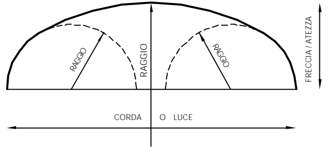
ARCO A SESTO POLICENTRICO
